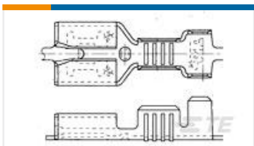
TE Part #100605-7 250 FASTON,REC.,14-17AWG,TPS
