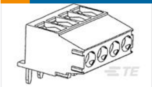
TE Part #1-284414-1 TERM-BLOK 900 PCB 11 POS 3,5
