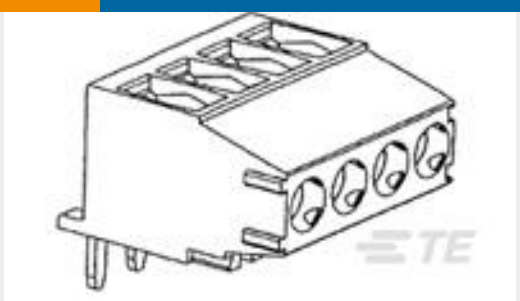
TE Part #1-284414-2 TERM-BLOK 900 PCB 12 POS 3,5
