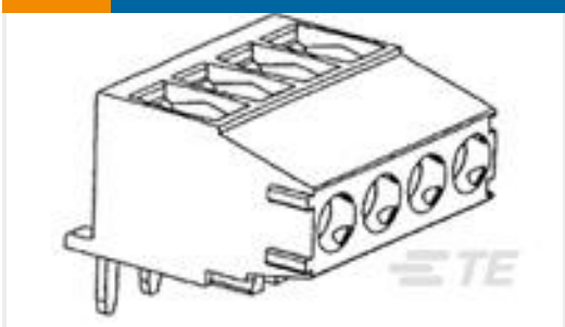
TE Part #1-284414-0 TERM-BLOK 900 PCB 10 POS 3,5
