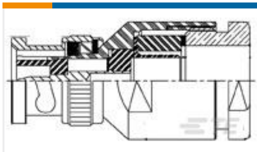
TE Part #1-1478404-0 BNC Str Plg PS 75Ohm Silver RG59B /U, 62A
