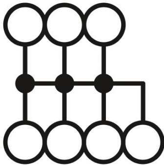
电路图
