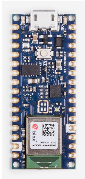
ARDUINO Nano 33 BLE (ABX00030/ ABX00034)
