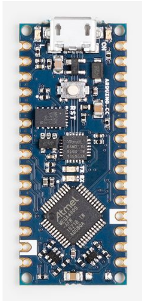
ARDUINO Nano Every (ABX00033/ ABX00028)
