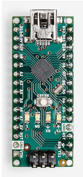
ARDUINO Nano (A000005)
