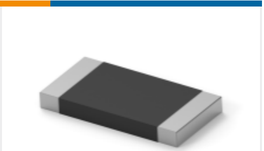
TE Part #3-2176230-8 3522 1K0 5% 3W
