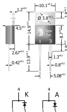
Dimensions - Maße [mm]
