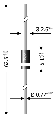
Dimensions - Maße [mm]
