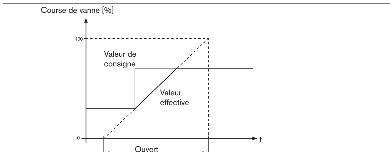
Fig. 41 : Diagramme X.TIME
