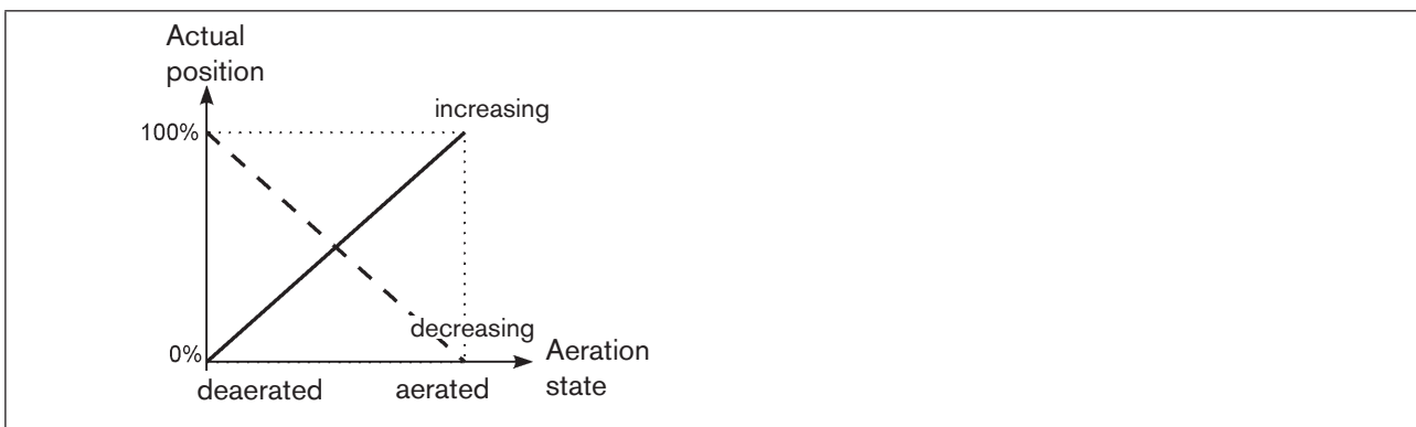
Fig. 35: DIR.ACTUATOR graph
