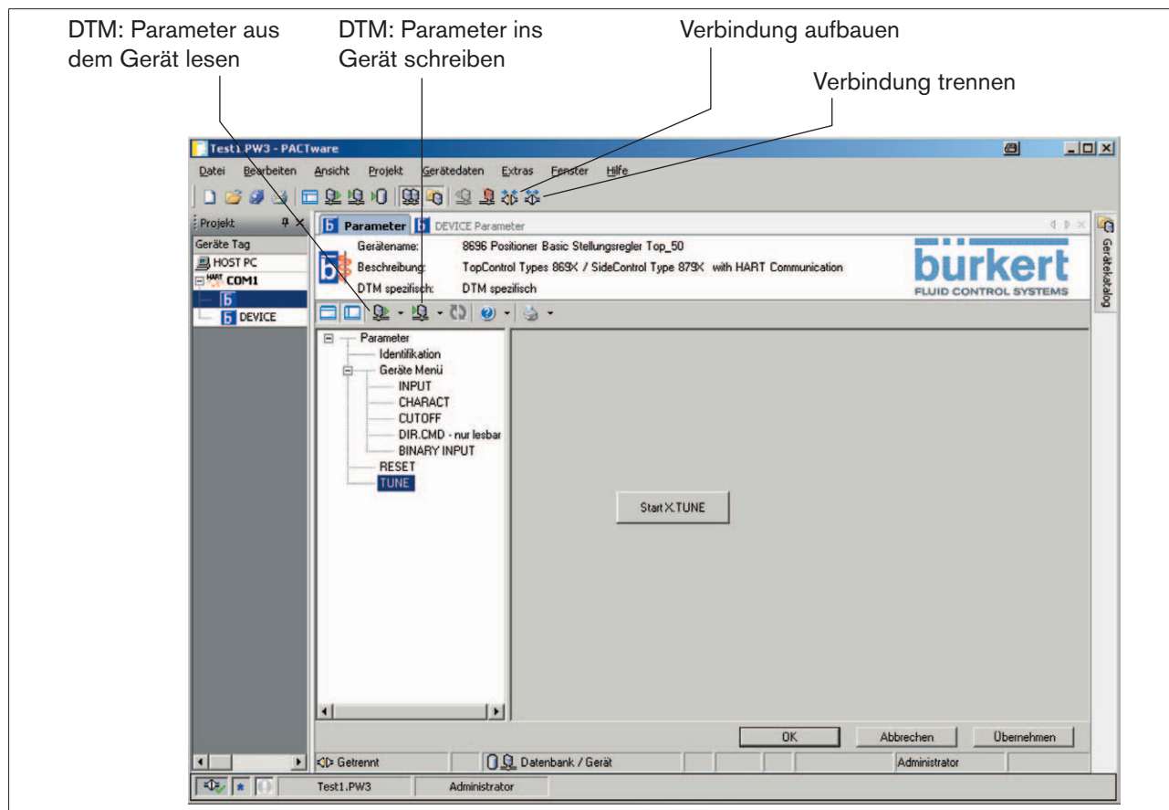
Bild 21: Parameter übertragen
