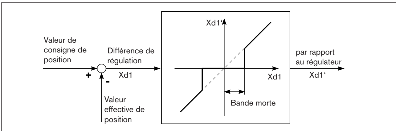
Fig. 43 : Diagramme X.CONTROL
