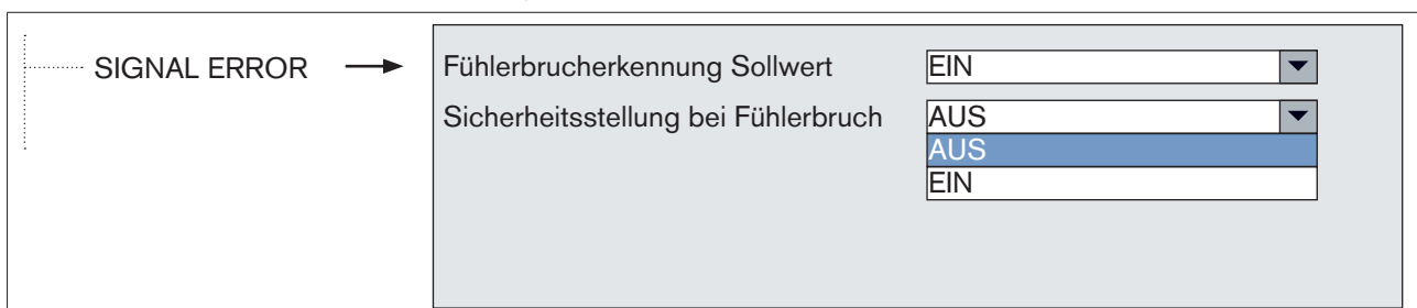
Bild 46: Funktion SIGNAL ERROR -2
