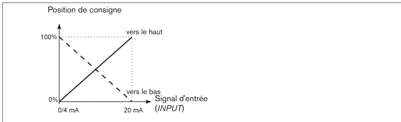
Fig. 31 : Diagramme DIR.CMD
