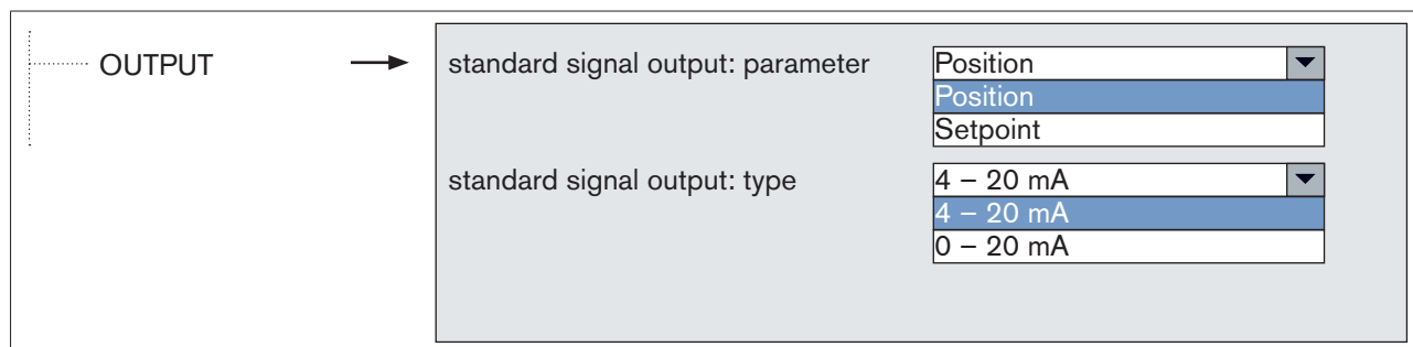
Fig. 48: OUTPUT function
