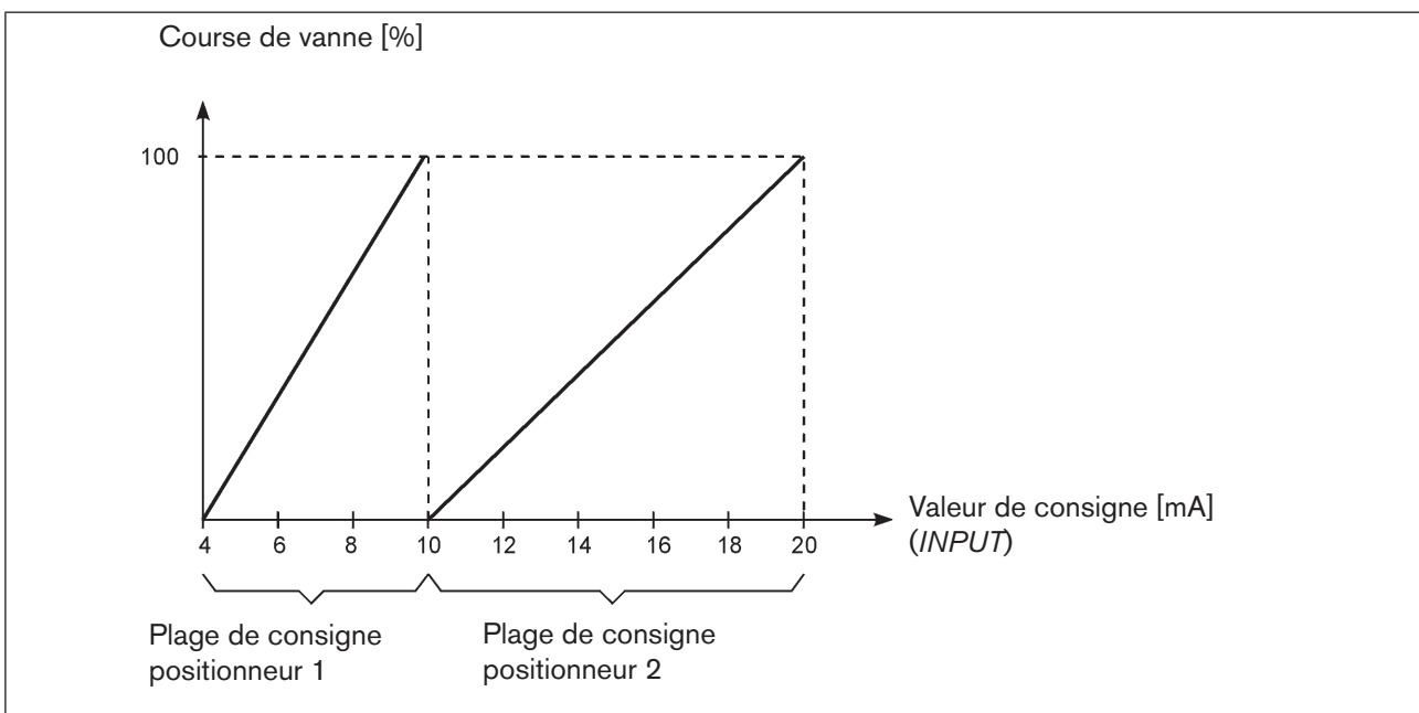
Fig. 37 : Diagramme SPLITRANGE
