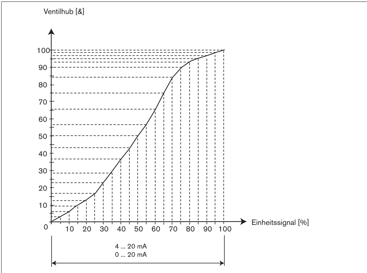
Bild 27: Beispiel einer programmierten Kennlinie
