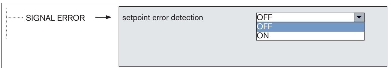
Fig. 45 : Fonction SIGNAL ERROR -1
