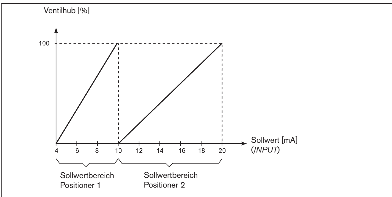
Bild 37: Diagramm SPLITRANGE
