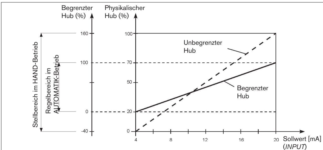
Bild 39: Diagramm X.LIMIT
