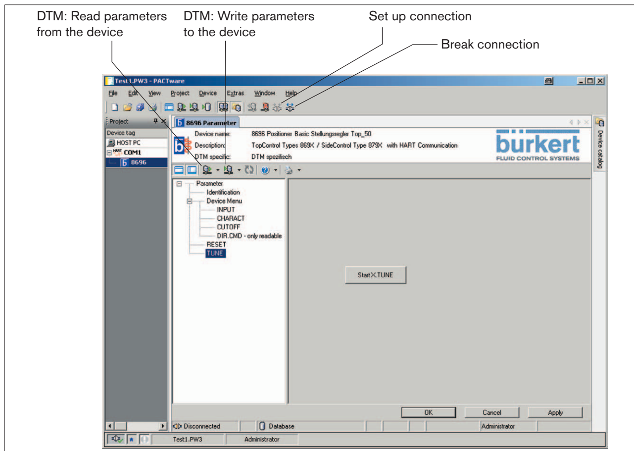
Fig. 21: Transferring parameters
