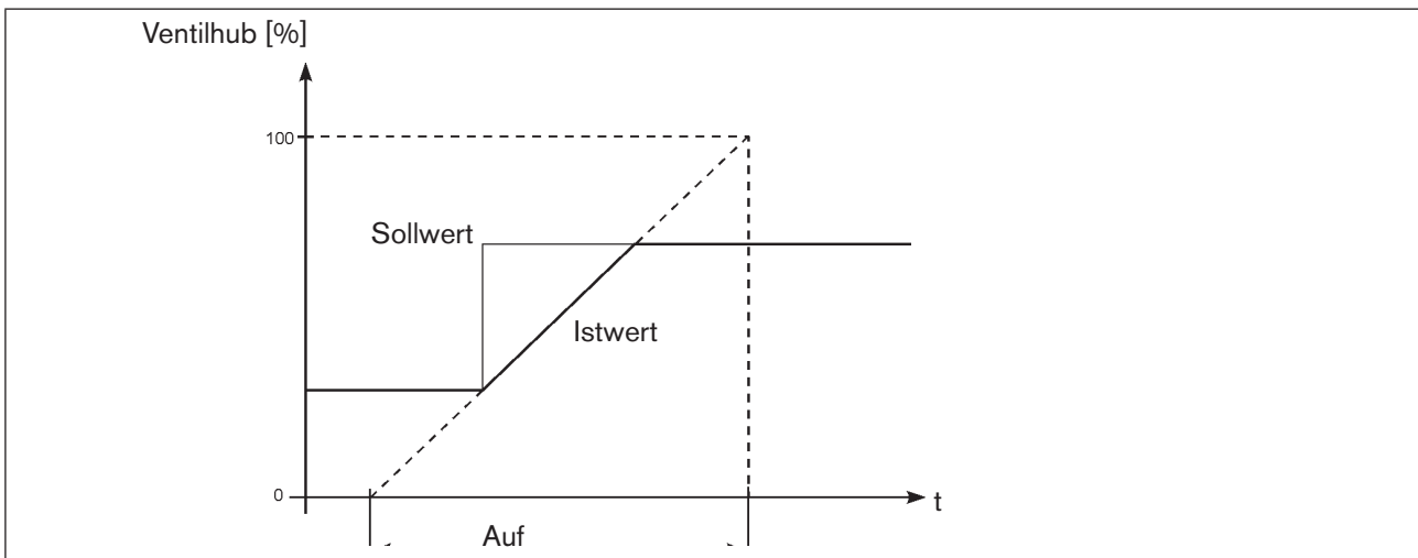
Bild 41: Diagramm X.TIME
