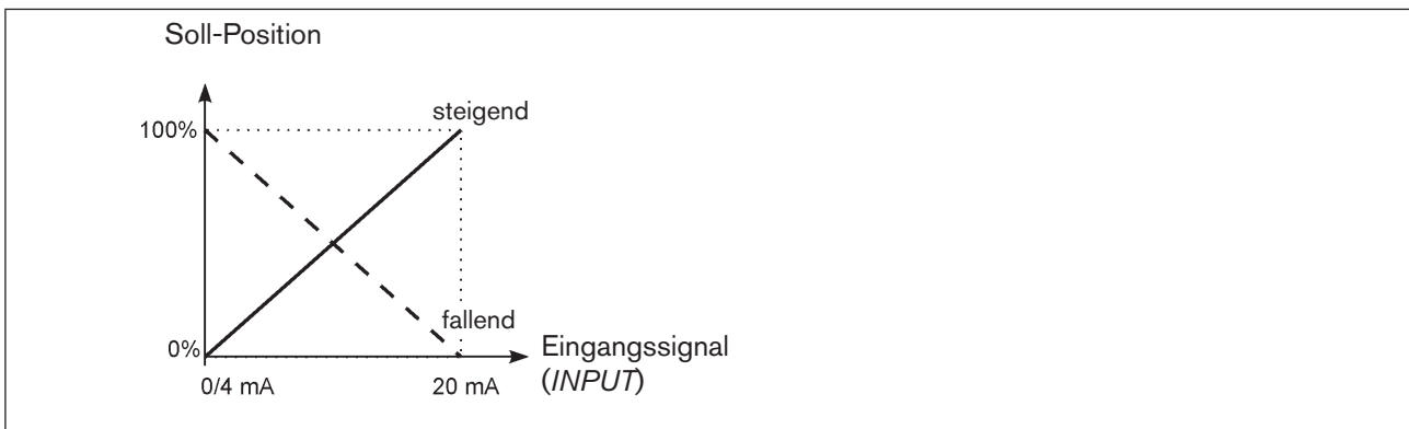
Bild 31: Diagramm DIR.CMD
