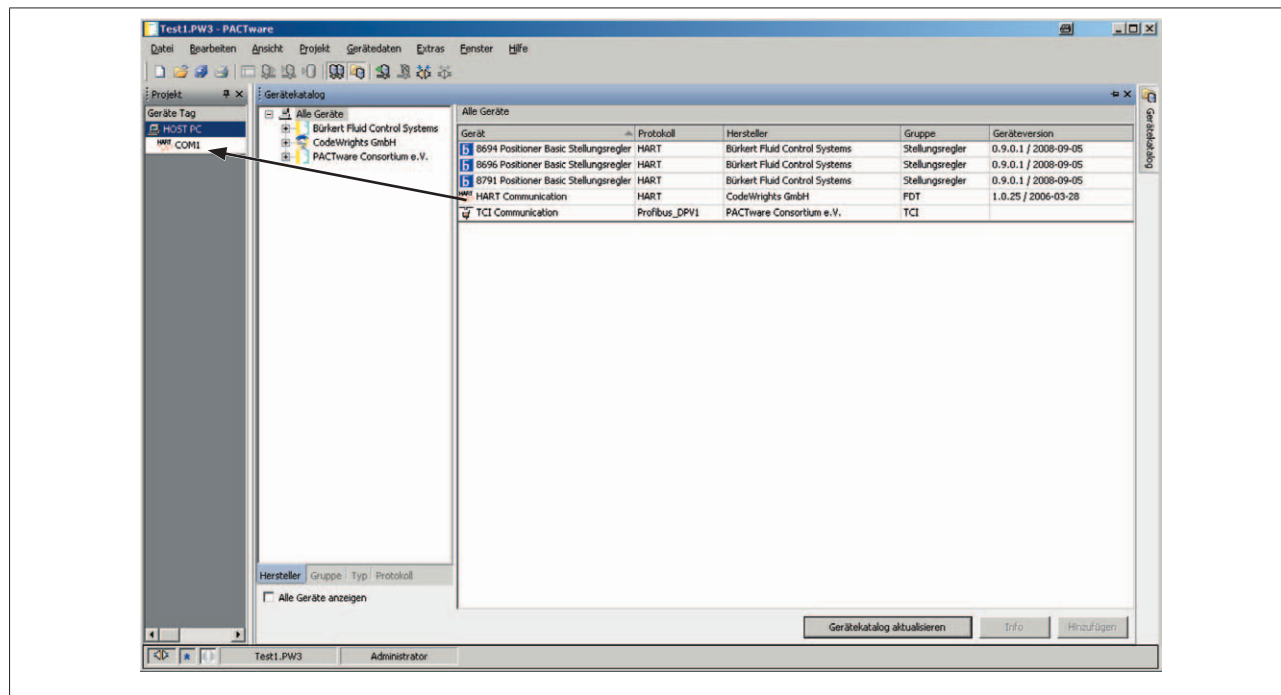
Bild 12: HART-Kommunikations-DTM einbinden
