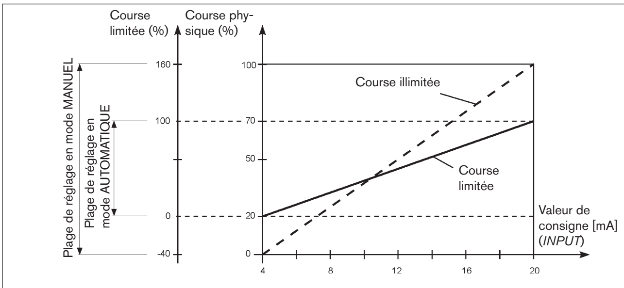
Fig. 39 : Diagramme X.LIMIT
