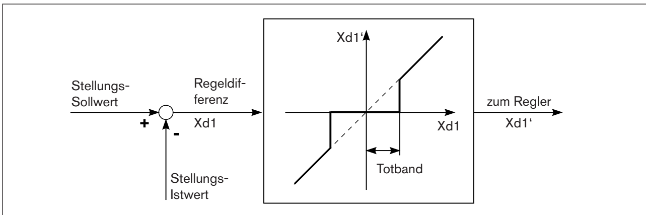
Bild 43: Diagramm X.CONTROL
