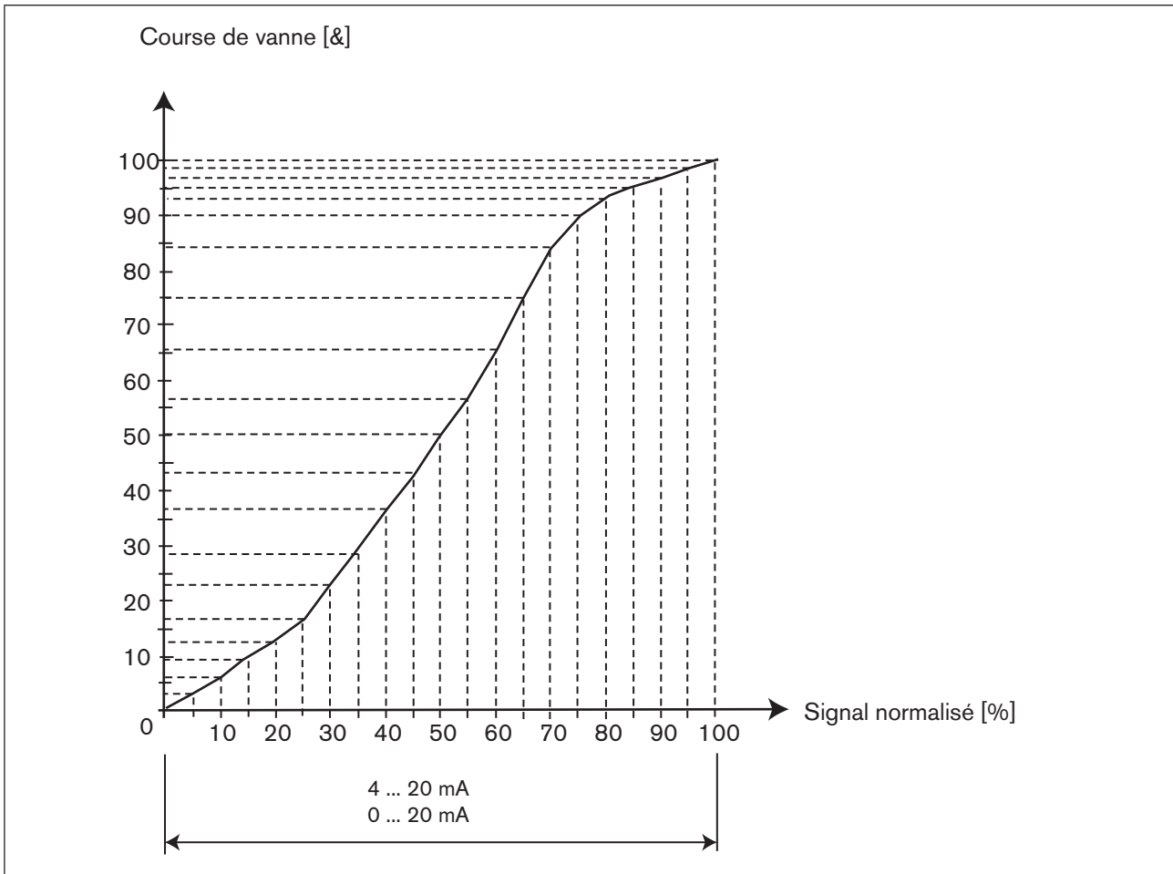
Fig. 27 : Exemple d'une caractéristique programmée
