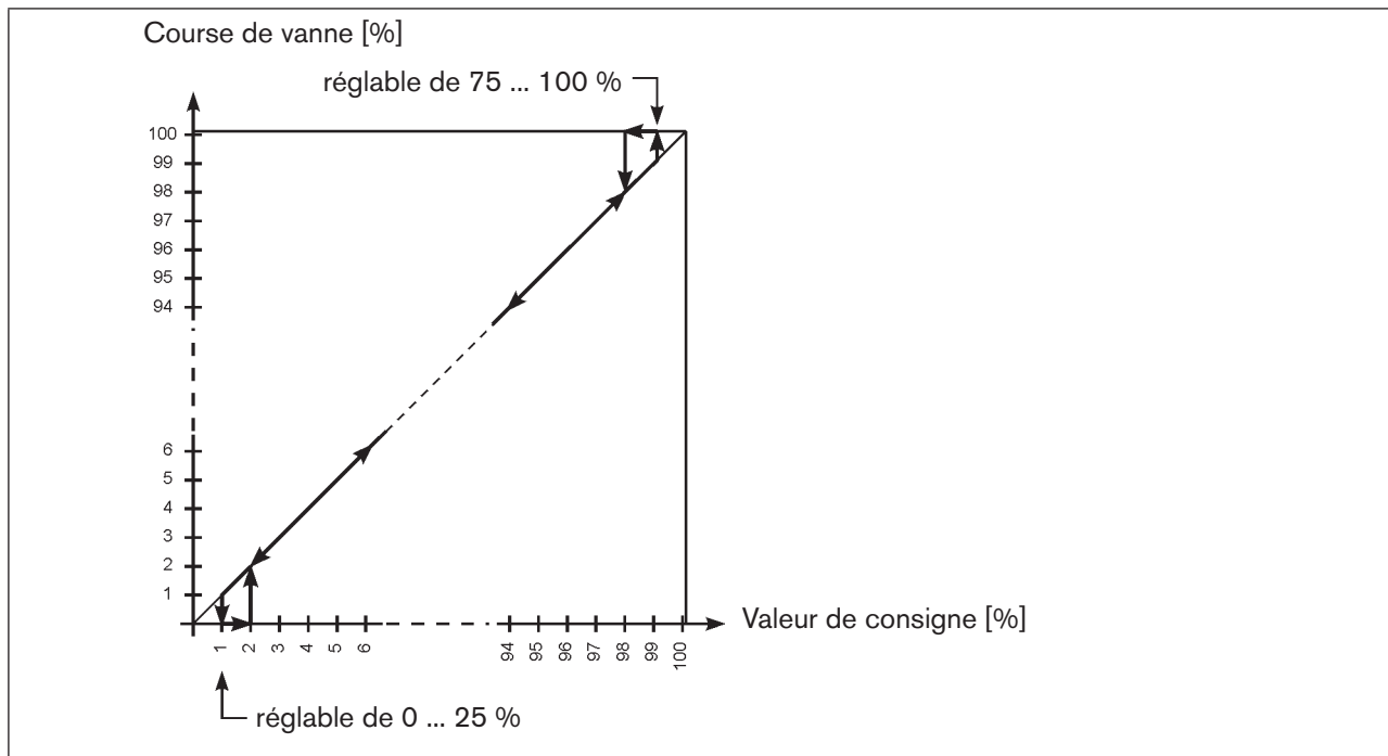
Fig. 29 : Diagramme CUTOFF
