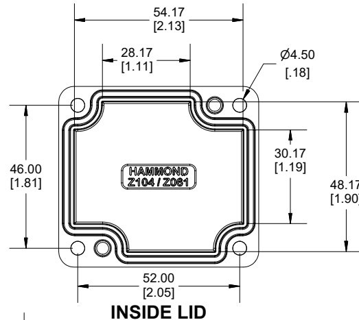
INSIDE LID
