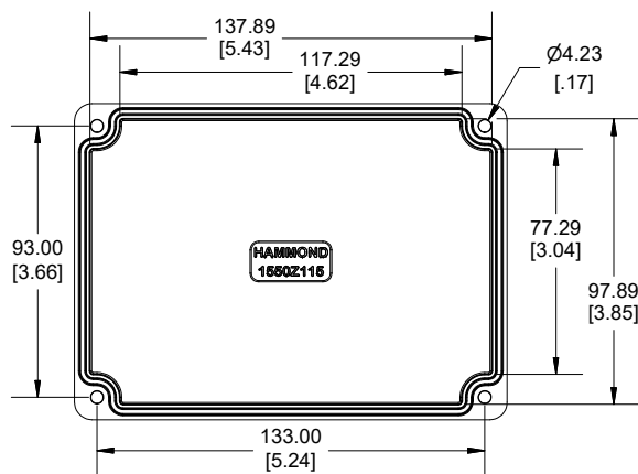
INSIDE LID
