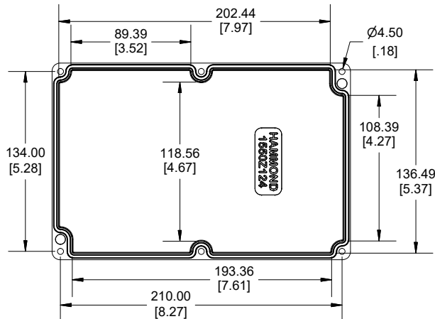
INSIDE LID
