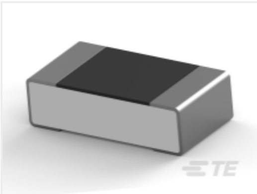
TE Part #5-2176367-6 RQ 0603 17K4 0.1% 10PPM 1K RL
