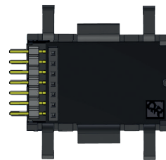
Abb.: Ausgangsbussverbinder für das Übergabemodul 800-CON-RJ45 am Ausgang einer Messgeräte- und Modulreihe.
