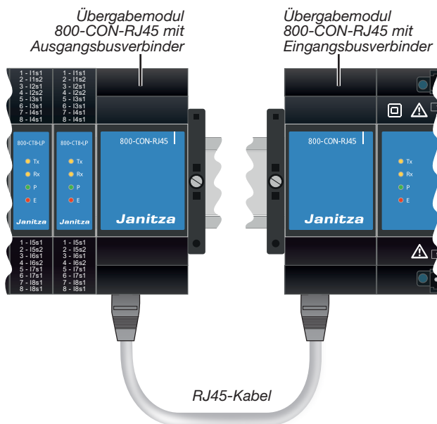
Abb.-Beispiel Messgeräte- und Modultopologie: RJ45-Verkabelung der Übergabemodule mit Aus- und Eingangsbusverbindern.
