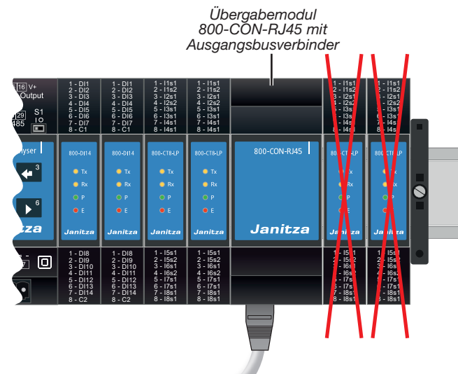
Abb.-Beispiel Messgeräte- und Modultopologie: Keine Weiterleitung der JanBus-Kommunikation bei Übergabemodulen mit Ausgangsbusverbindern.
