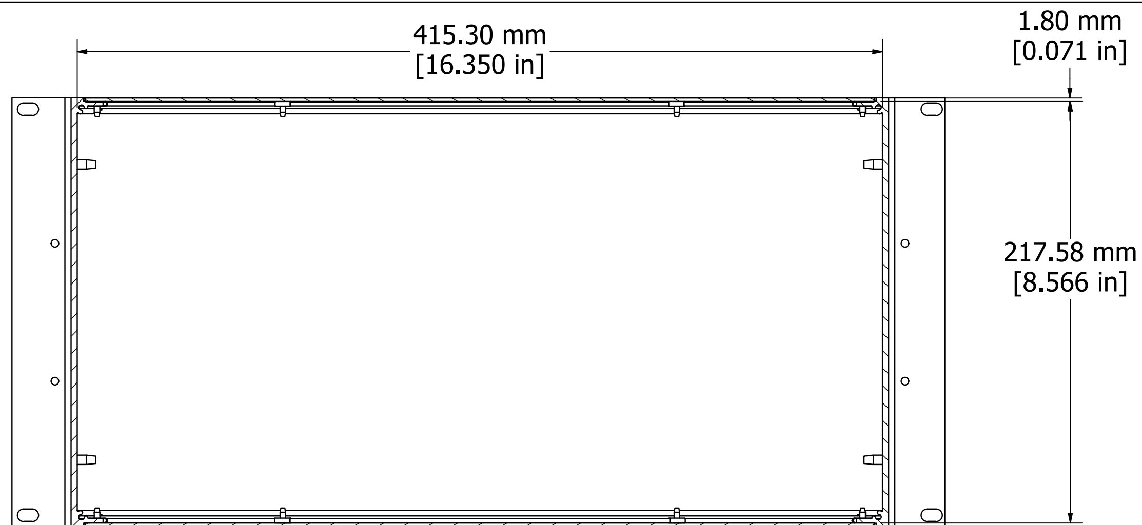
SECTION A-A
