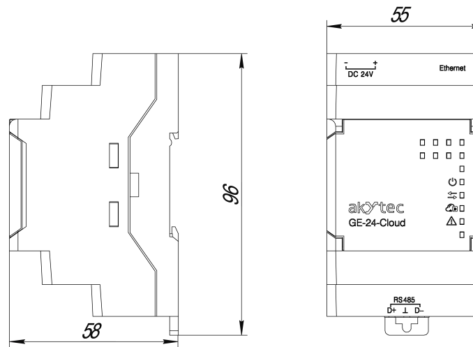
Fig. 1 Dimensions
