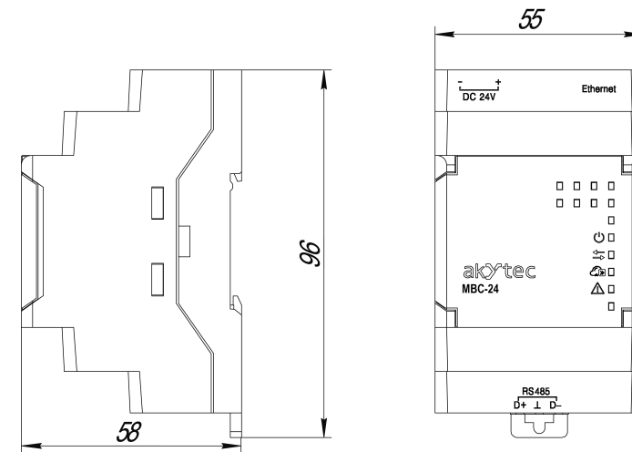
Fig. 1 Dimensions
