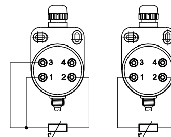
Fig. 1 Wiring
