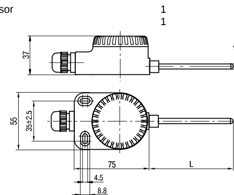
Fig. 2 Dimensions
