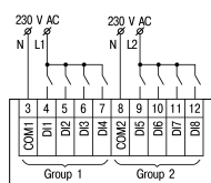
Fig. 5 – Digital inputs wiring (230 V AC)
