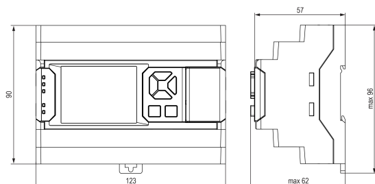
Fig. 1 – Dimensions
