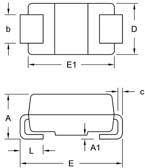
DO-214AC (SMA)
