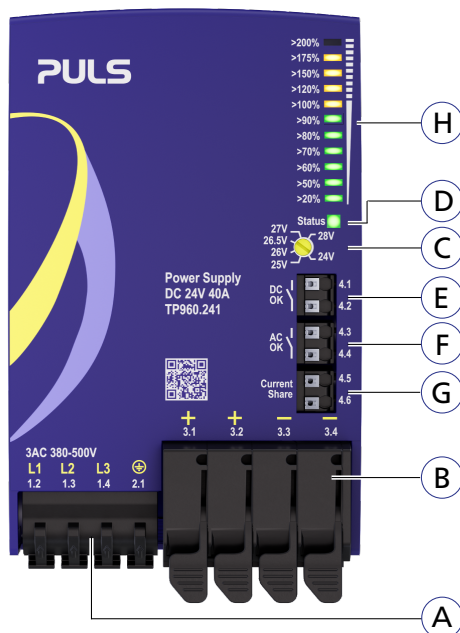
Fig. 18-1: Front side
