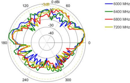
Elevation 2: 6000 – 7200 MHz
