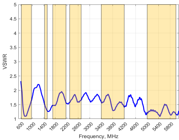
VSWR
