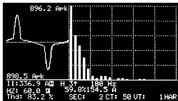
(Corriente distorsionada con armónicos)
