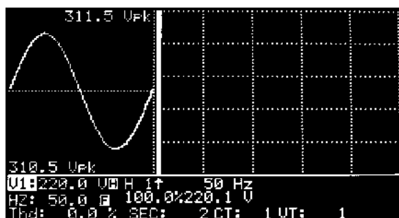
(Tensión normal sin distorsión y armónicos)
