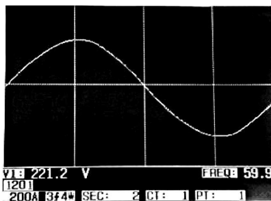
Fig. 5-9b: Formas de onda - Pantalla 2
