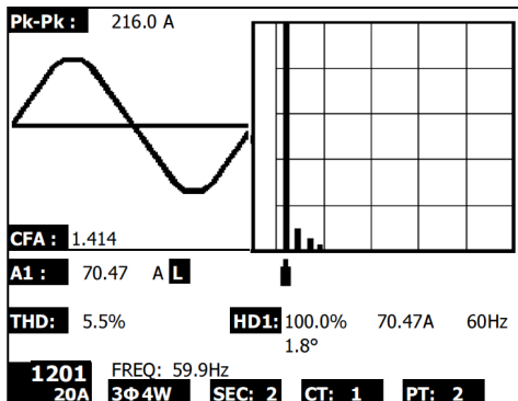
Fig. 5-7b: Armónicas - Pantalla 2
