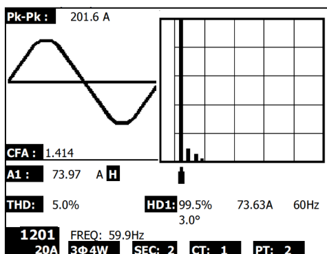
Fig. 5-7d: Armónicas - Pantalla 4
