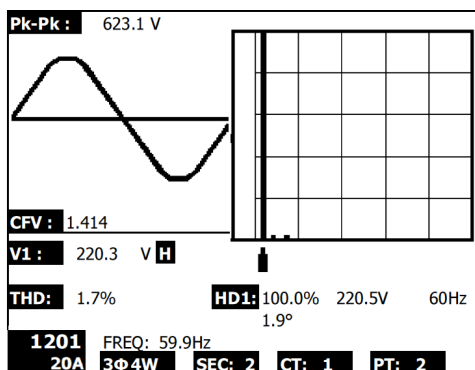
Fig. 5-7d: Armónicas - Pantalla 4
