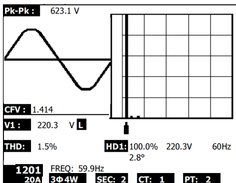
Fig. 5-7a: Armónicas - Pantalla 1
