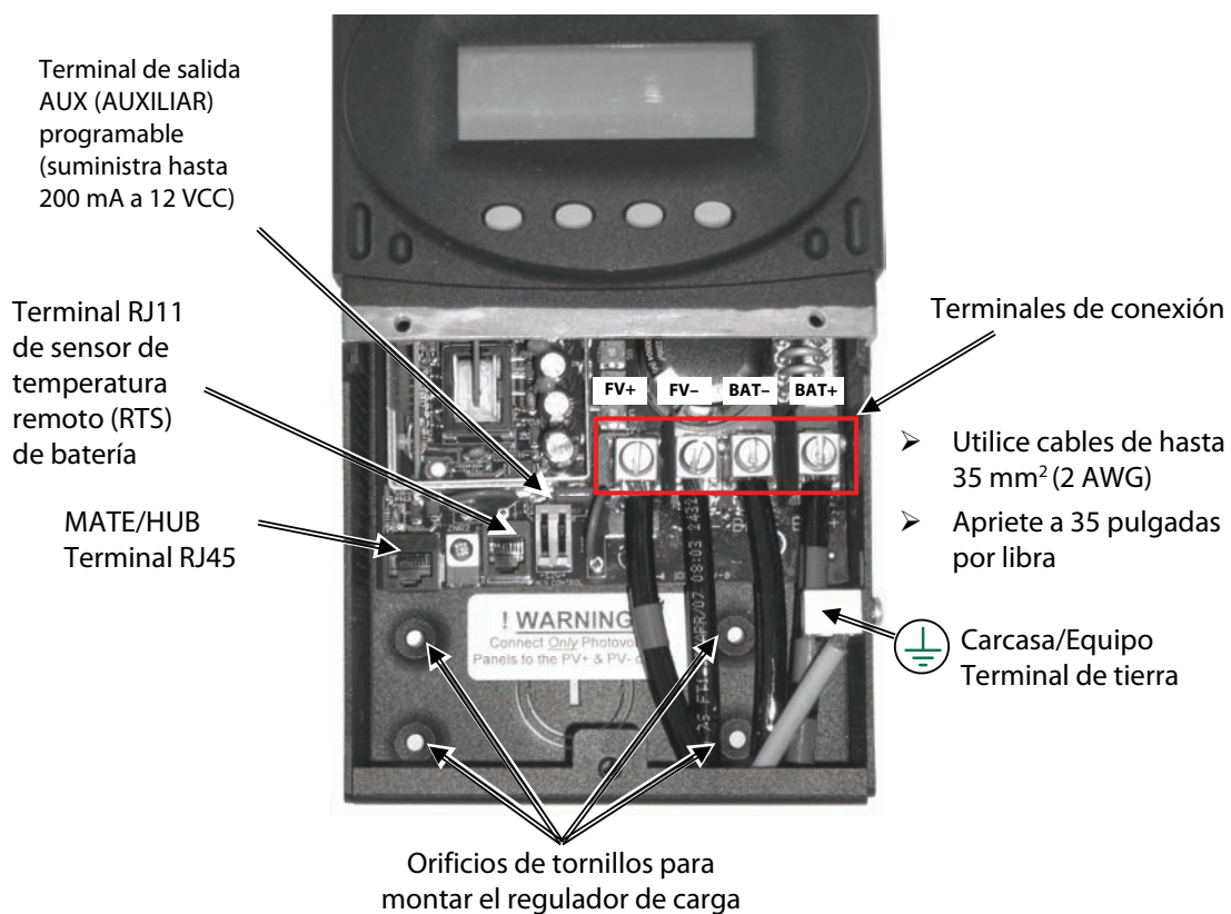
Figura 3 Compartimento del cableado
