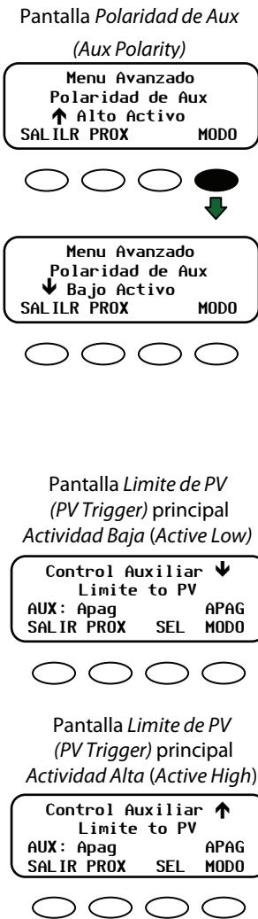
Figura 45 Pantalla Polaridad de auxiliar (Aux Polarity)
