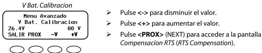
Figura 42 Calibración del voltaje de la batería (Vbatt Calibration)
