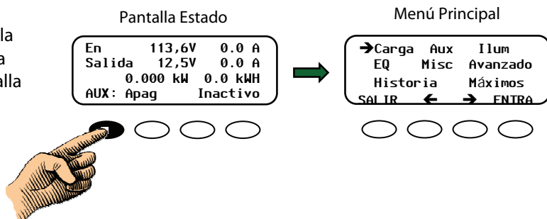
Figura 12 Acceso al Menú Principal
