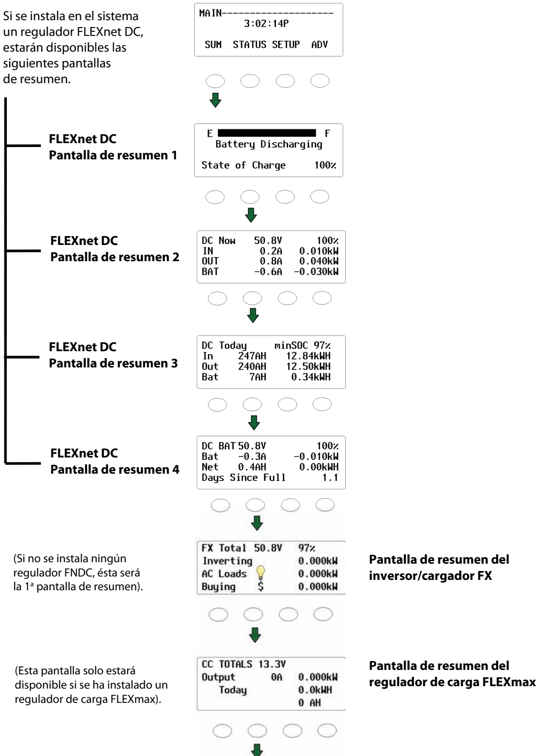
Figura 64 Mapa de menús de pantallas de resumen
