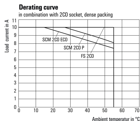
Curva de deriva Relé combinado con base
