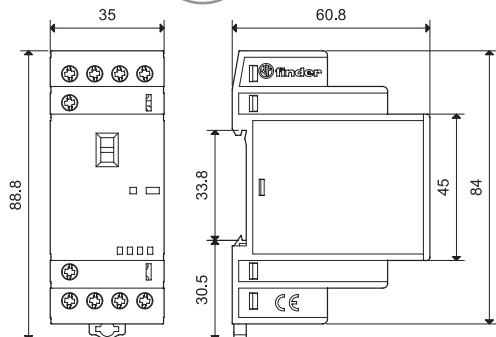
Tipo 22.44/22.64 Borne de jaula
