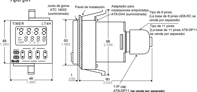
Tipo pin
