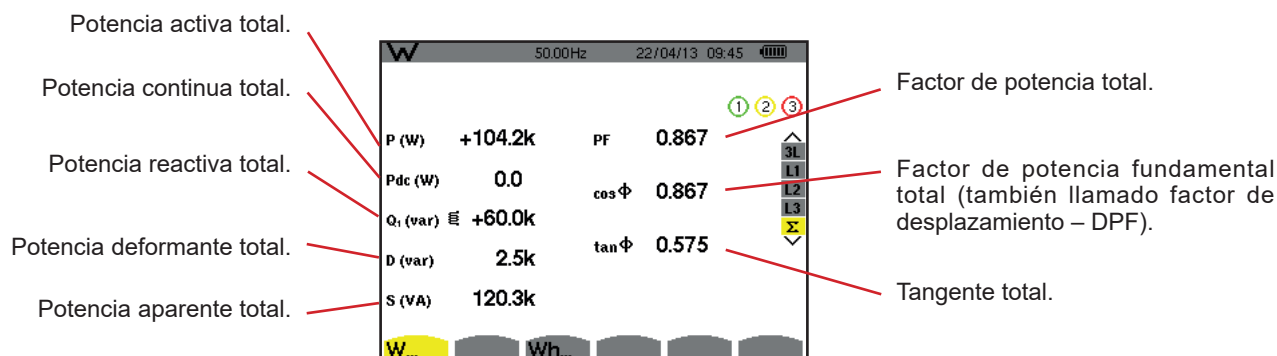
Figura 115: la pantalla de visualización de las potencias y magnitudes totales asociadas en \Sigma
