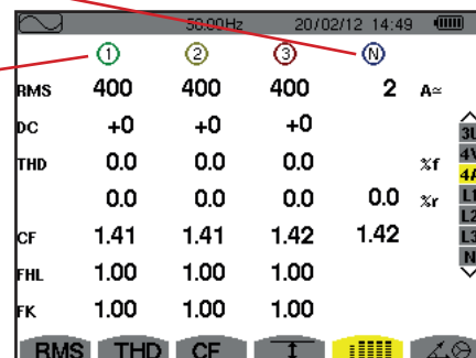
Figura 80: la pantalla de visualización simultánea en 4A
