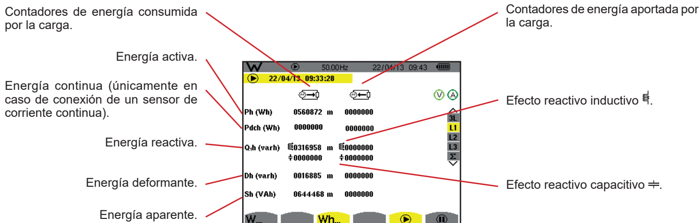
Figura 114: la pantalla de visualización de las energías consumidas y aportadas en L1
