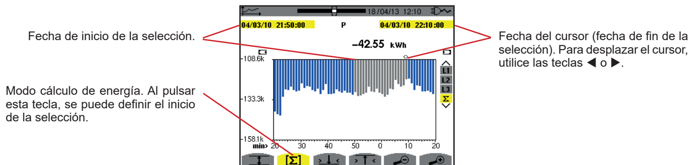
Figura 101: Ph(\Sigma) sin MIN-AVG-MAX
