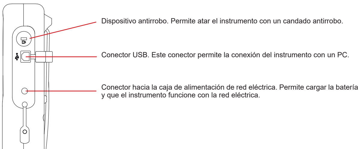
Figura 4: los conectores laterales
