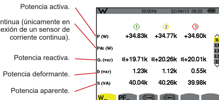
Figura 109: la pantalla de las potencias en 3L
