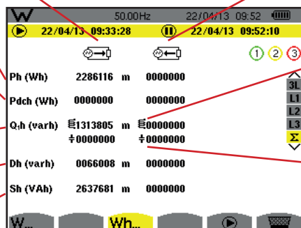
Figura 116: la pantalla de visualización de las energías consumidas y aportadas totales en \Sigma
