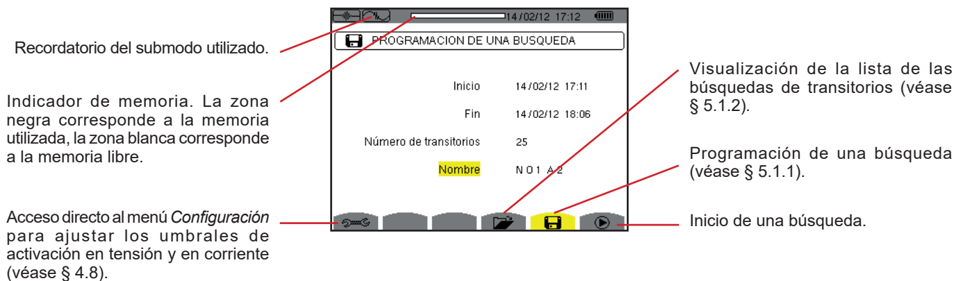
Figura 38: la pantalla Programación de una búsqueda en modo transitorios
