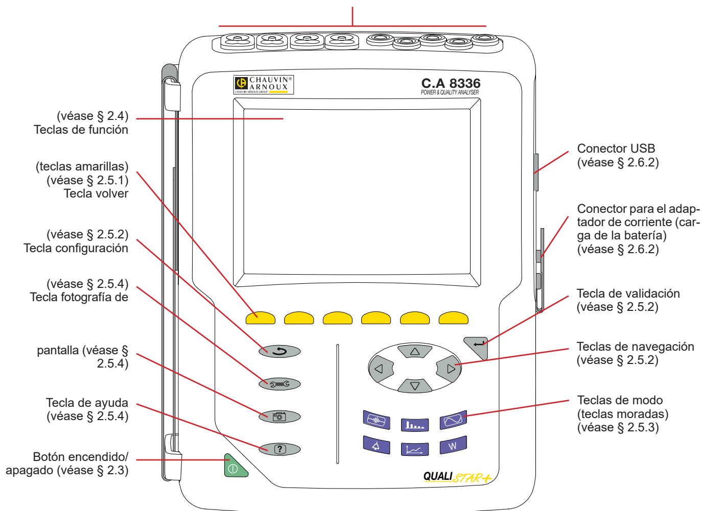
Figura 1: vista general del Qualistar+
