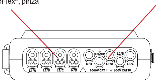
Figura 3: los bornes de conexión
