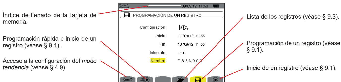
Figura 88: la pantalla del modo tendencia
