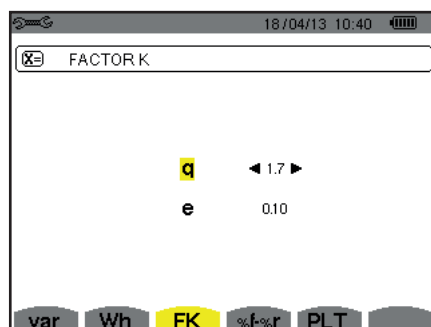
Figura 22: el menú Selección de los coeficientes de cálculo del factor K
