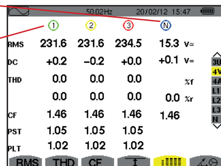
Figura 79: la pantalla de visualización simultánea en 4V
