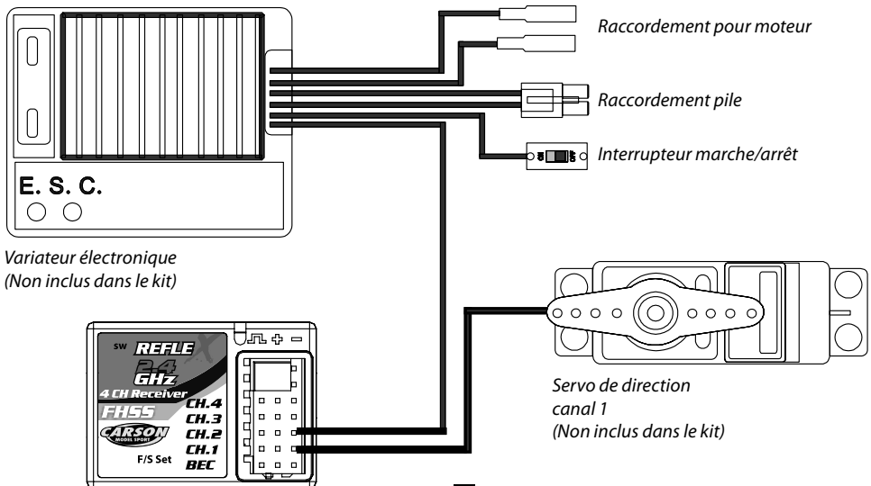
Récepteur
