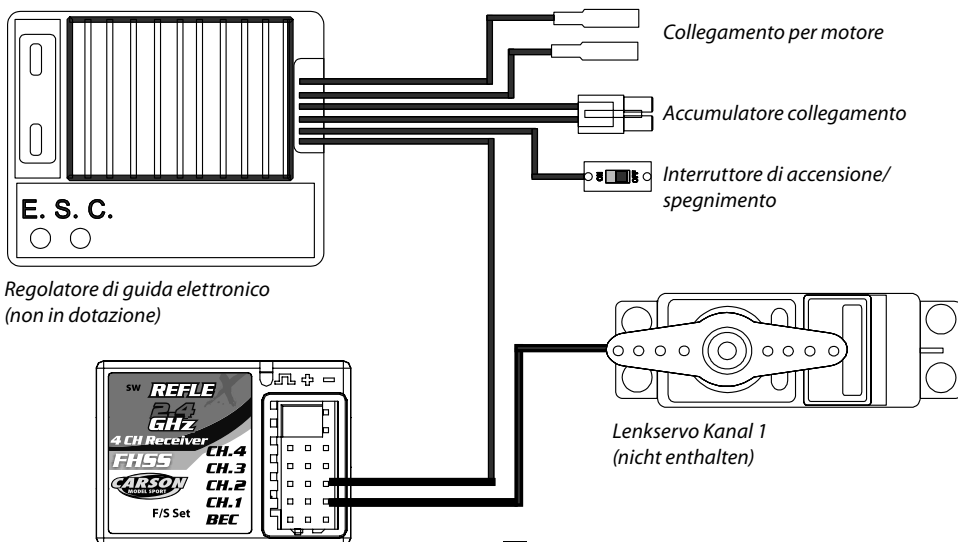
Ricevitore Non è necessario collegare un'alimentazione separata per il ricevitore!
