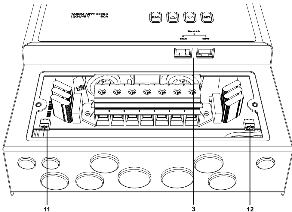
Fig. 4: Vista general de las conexiones adicionales MPPT 6000-S
