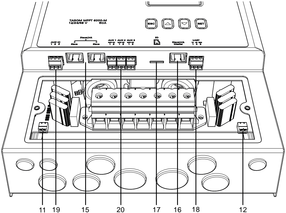
Fig. 3: Vista general de las conexiones adicionales MPPT 6000-M
