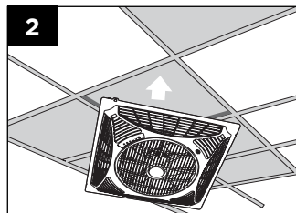
2. Coloque el ventilador de techo dentro del falso techo.
