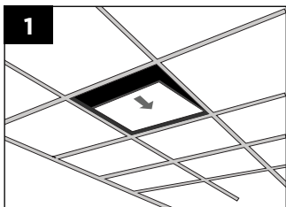
1. Retire una de las placas del falso techo.
