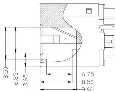
Dibujo acotado
