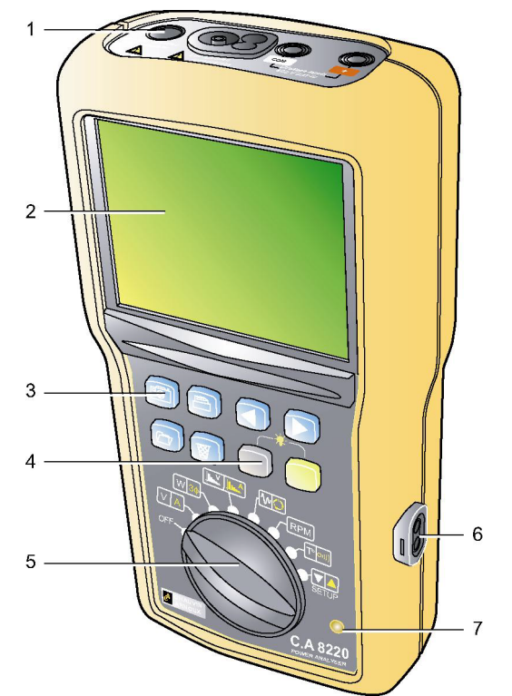
Figura 1: Vista general del C.A 8220.
