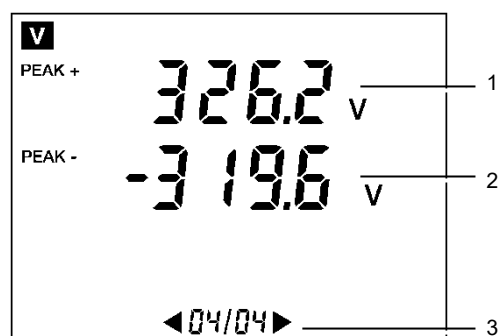
Figura 12: Ejemplo de visualización de la página 4/4.
