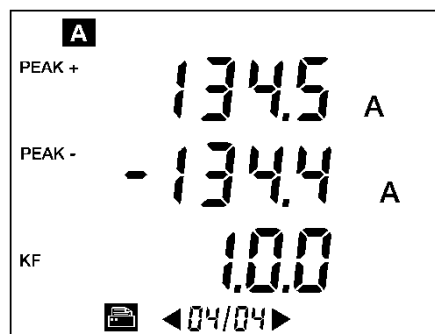
Figura 58: El icono de impresora parpadea durante la transferencia de informaciones hacia la impresora térmica de serie.
