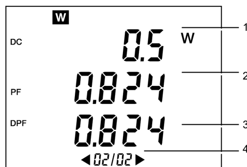
Figura 2: Ejemplo de visualización de la página 2/2.
