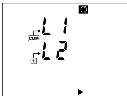
Figura 31: El C.A. 8220 está listo para la primera medida de determinación del orden de fases.
