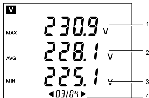
Figura 11: Ejemplo de visualización de la página 3/4.
