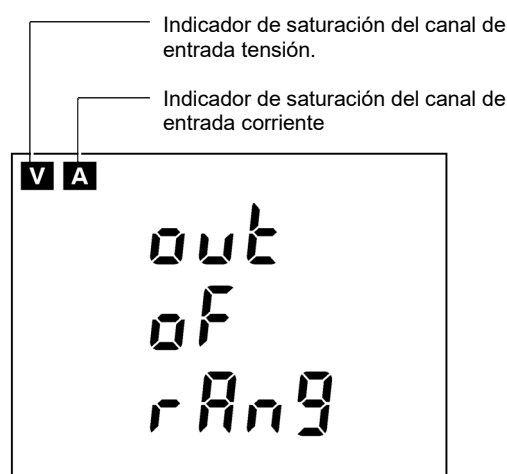
Figure 73: Indicadores de canales de entrada saturados.
