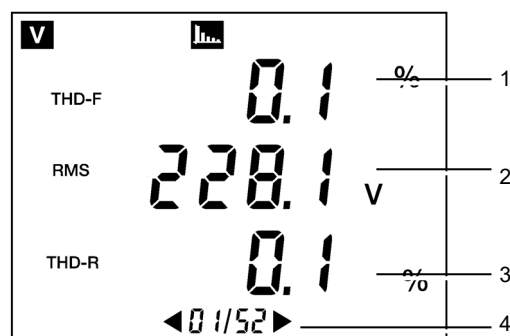
Figura 20: Ejemplo de visualización de la página 1/52.
