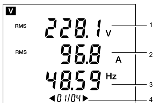
Figura 9 : Ejemplo de visualización de la página 1/4.
