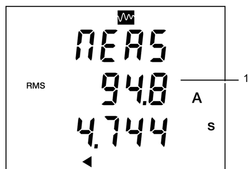
Figura 29: El cronómetro (parte inferior de la pantalla) está activo siempre que no se alcance el umbral de corriente baja.
