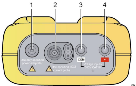
Figura 2: Los terminales en la parte superior.
