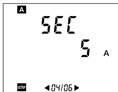
Figura 45: Visualización del parámetro relativo a la corriente eficaz secundaria del transformador de intensidad.
