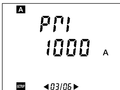
Figura 44: Visualización del parámetro relativo a la corriente eficaz primaria del transformador de intensidad.
