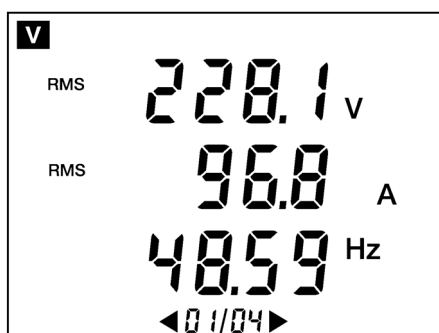
Figura 67: Ejemplo de tercera pantalla (función de la posición del interruptor de giro).
