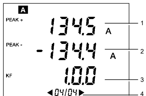
Figura 16: Ejemplo de visualización de la página 4/4.
