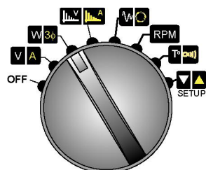
Figura 17: El interruptor de giro en la posición W 3Φ .
