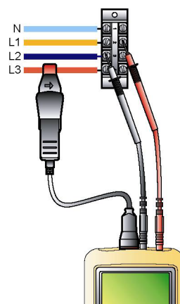
Figura 70: Conexión en red trifásica equilibrada. 006
