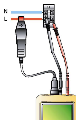
Figura 69: Conexión en red monofásica. 005
