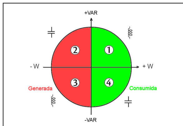
Figura 72: Representación de los 4 cuadrantes de potencia.
