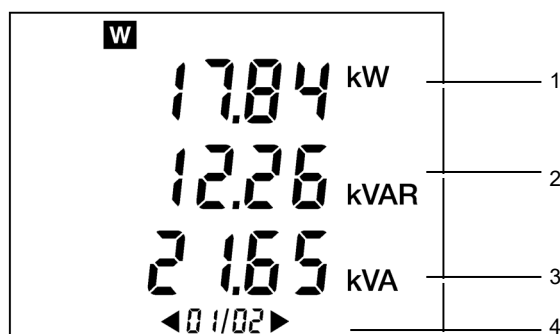
Figura 1: Ejemplo de visualización de la página 1/12.
