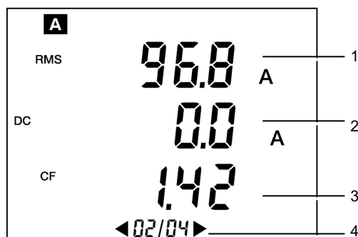
Figura 14: Ejemplo de visualización de la página 2/4.
