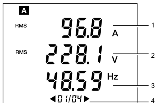
Figura 13: Ejemplo de visualización de la página 1/4.
