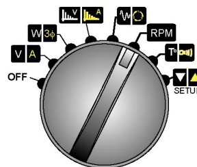
Figura 36: El interruptor de giro en la posición RPM .
