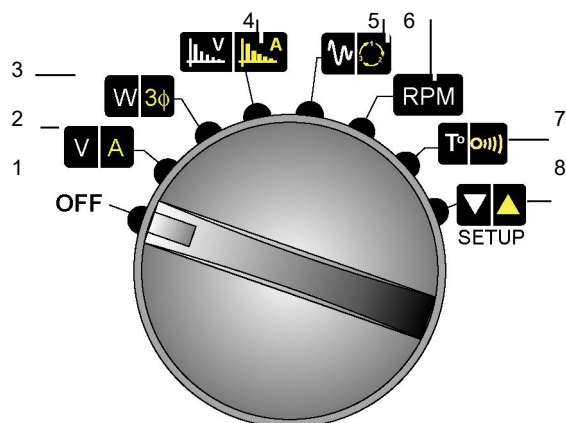
Figura 6: Vista de los modos accesibles desde el interruptor de giro.
