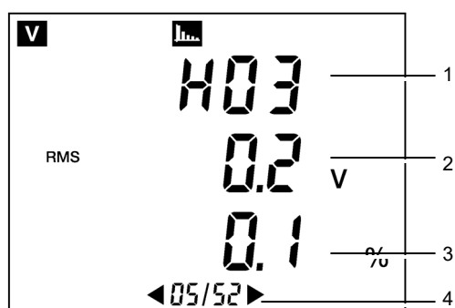
Figura 22: Ejemplo de visualización de la página 5/52.
