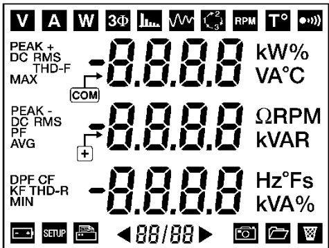
Figura 3: Segmentos que se visualizan.
