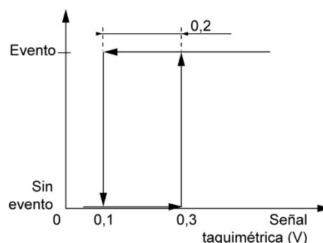
Figura 50: Funciones de determinación de evento.
