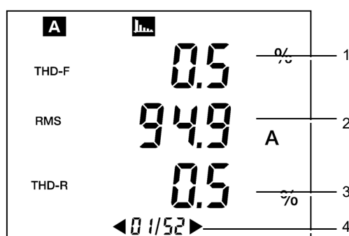
Figura 23: Ejemplo de visualización de la página 1/52.
