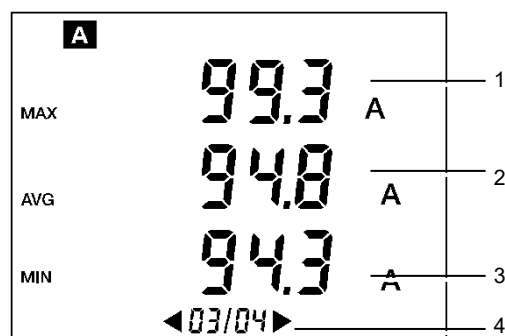
Figura 15: Ejemplo de visualización de la página 3/4.
