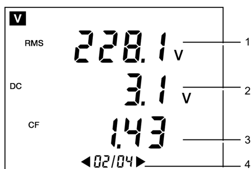
Figura 10: Ejemplo de visualización de la página 2/4.
