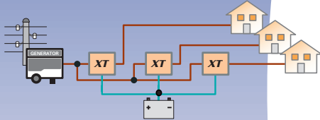
Centralizado
