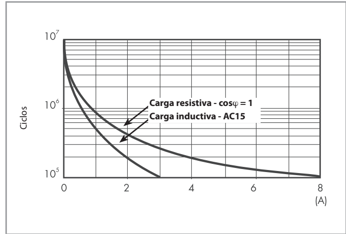
F 40.4 - Vida útil eléctrica (AC) en función de la carga Tipo 40.52 (página 4)
