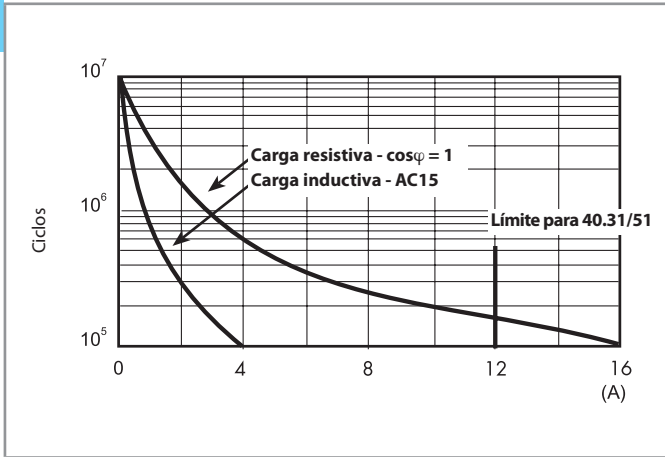
F 40.3 - Vida útil eléctrica (AC) en función de la carga Tipos 40.31/51/61 (página 4)
