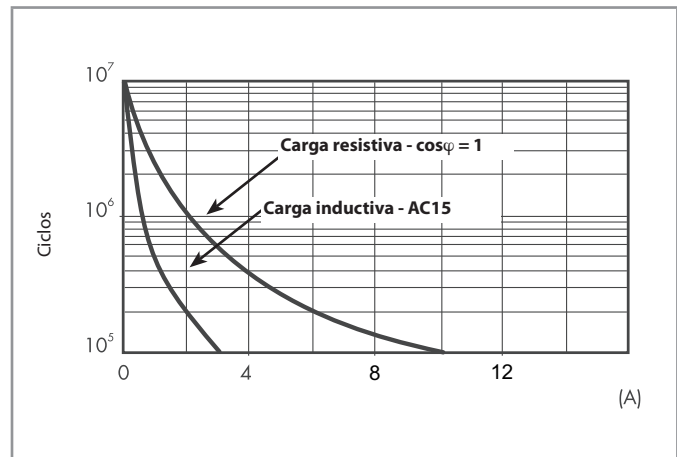
F 40.6 - Vida útil eléctrica (AC) en función de la carga Tipo 40.62 (página 5)
