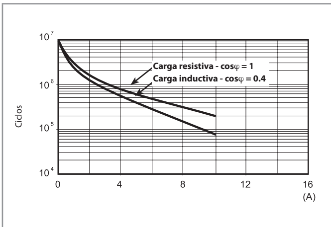
F 40.5 - Vida útil eléctrica (AC) en función de la carga Tipo 40.11 (página 5)
