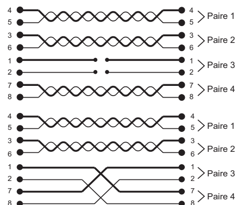
Ejemplos de esquemas de identificación de pares cortados y cruzados en los cables
