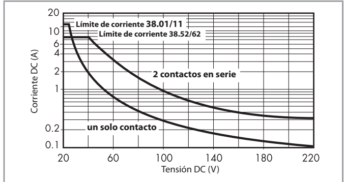
H 38 - Poder de corte para cargas en DC1, 1 contacto 16 A y 2 contactos 8 A
