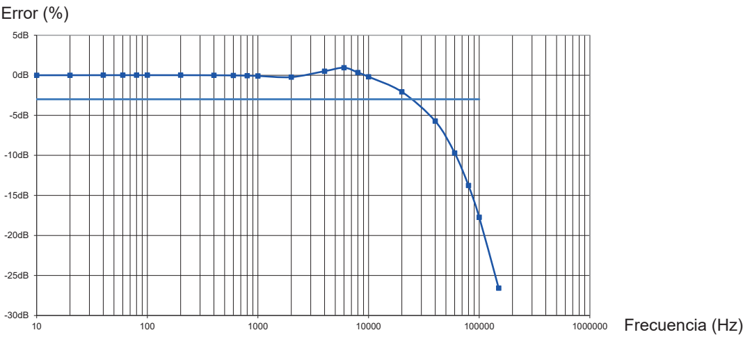
Curva típica del error en amplitud a 100 A en función de la frecuencia, I = 0,5 A, rango 1 V/A
