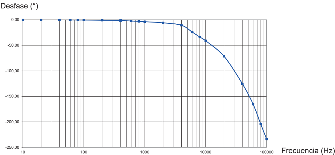
Curva típica del error de fase en función de la frecuencia, I = 0,5 A, rango 1 V/A
