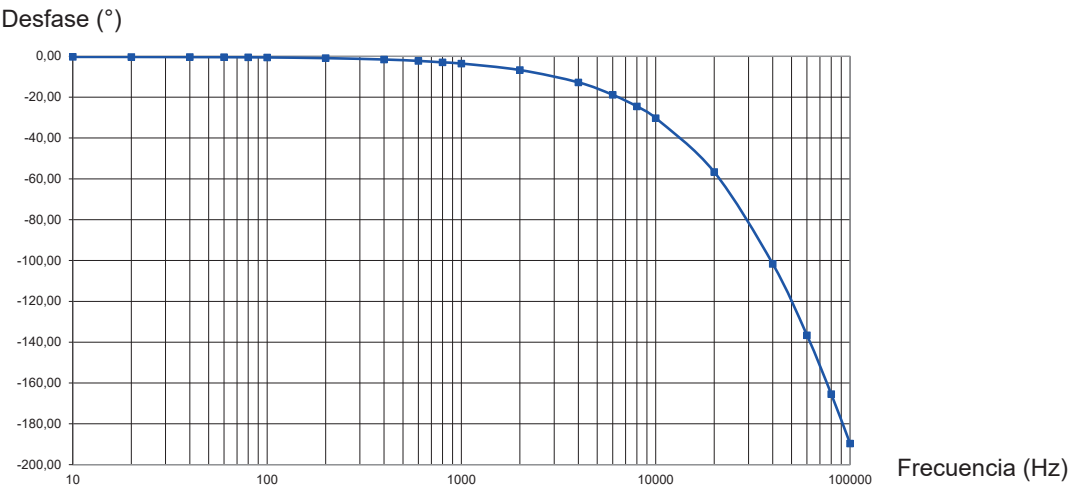
Curva típica del error de fase en función de la frecuencia, I = 1 A, rango 10 mV/A
