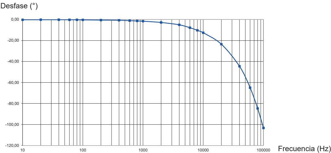
Curva típica del error de fase en función de la frecuencia, I = 1 A, rango 100 mV/A
