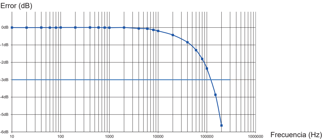
Curva típica del error en amplitud a 1 A en función de la frecuencia, rango 100 mV/A
