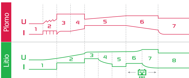
Curva de carga específica en 7 etapas sin vigilancia.
