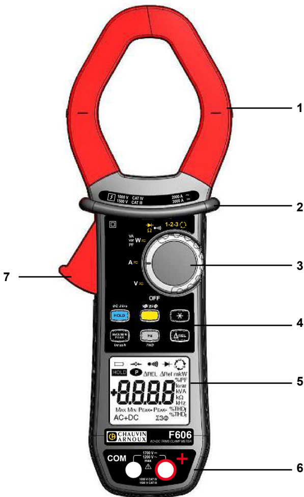
Figura 1 : la pinza multimétrica F606
