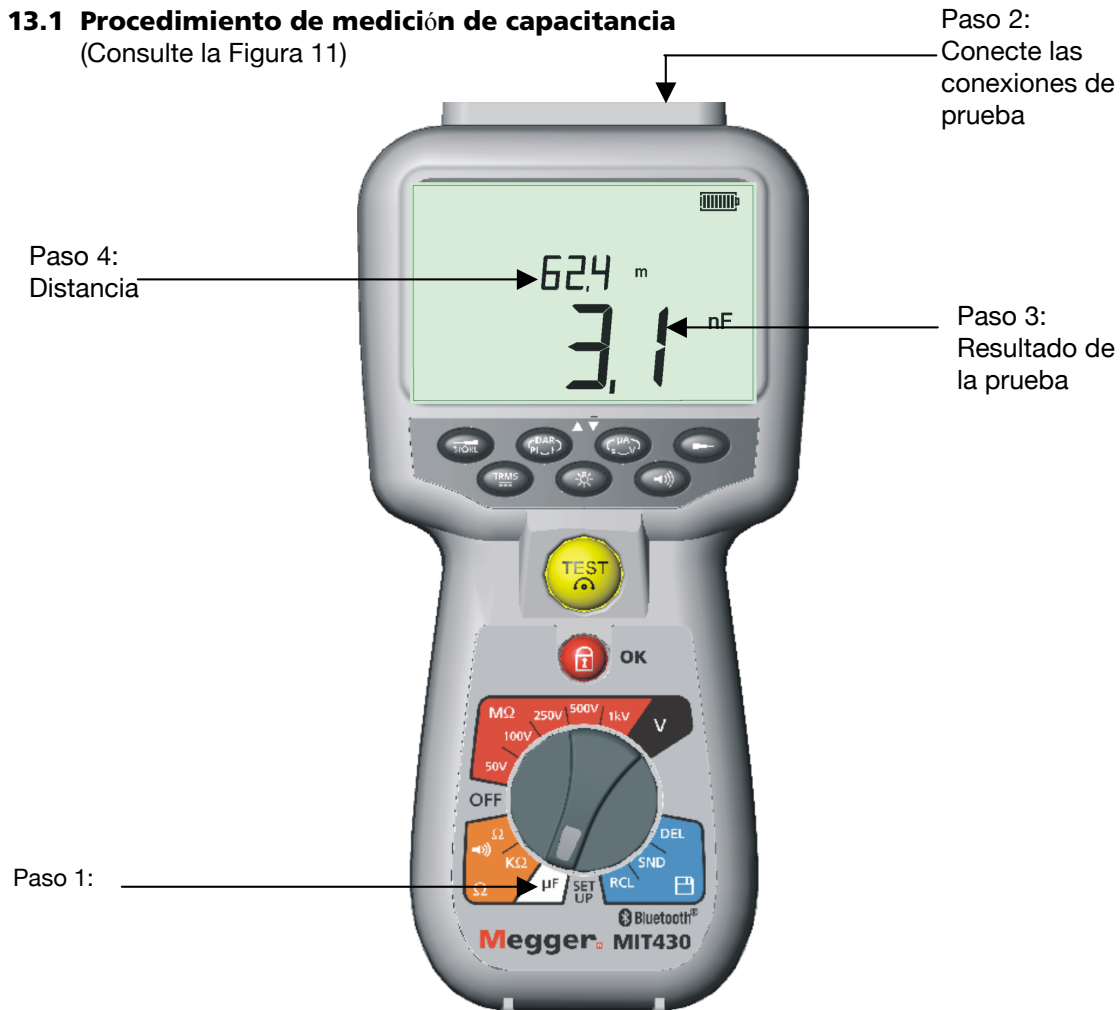
Figura 11, Rango de capacitancia
