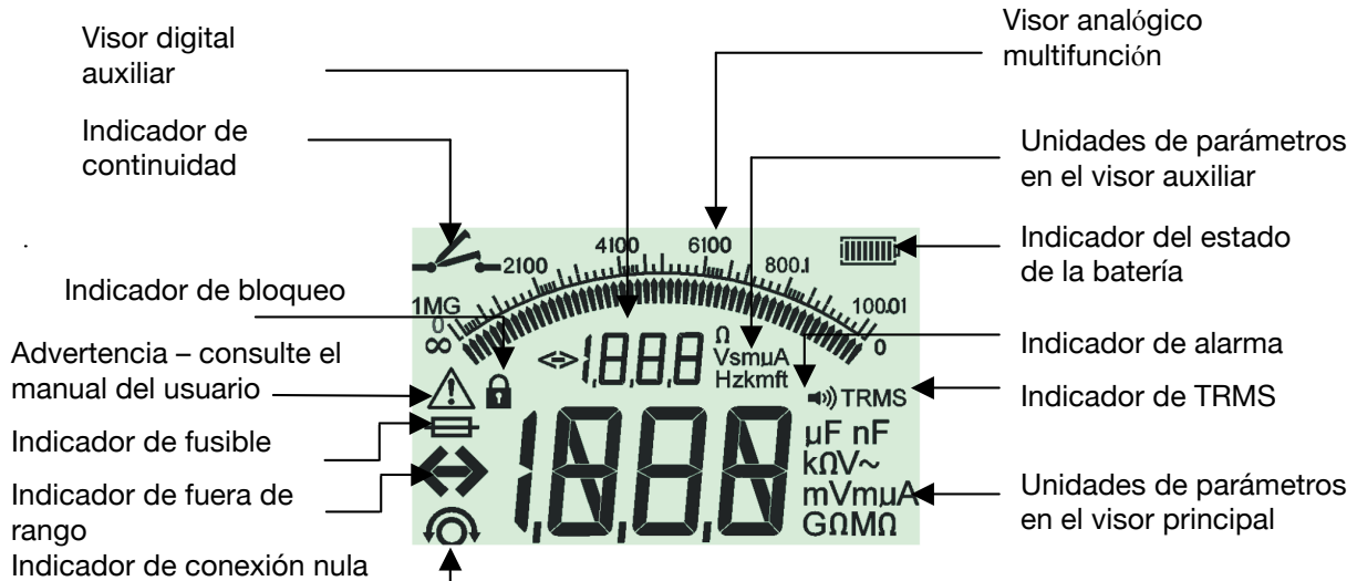
Figura 1, Visor de LCD
