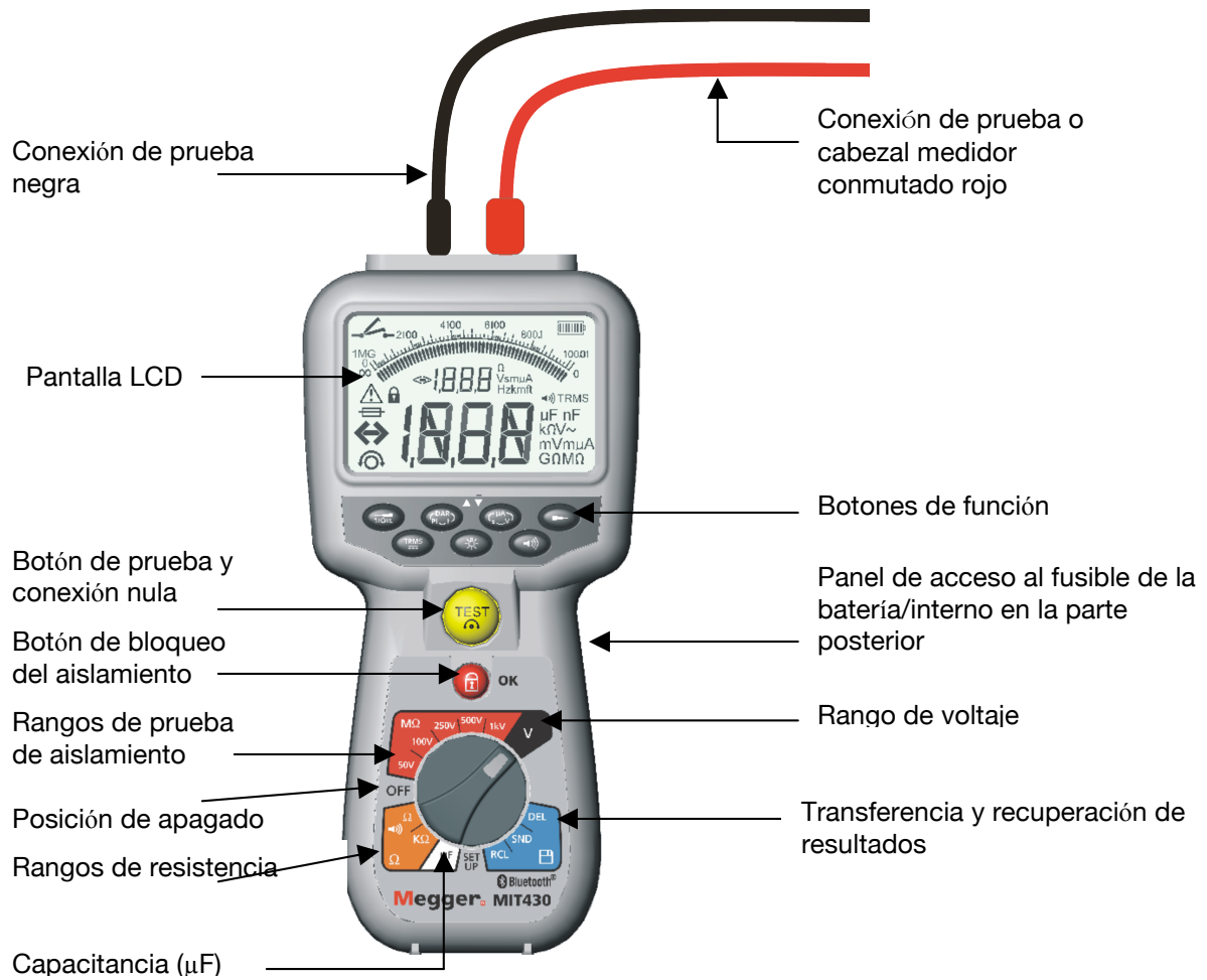
Características principales de la Figura 3 (Imagen de MIT430)
