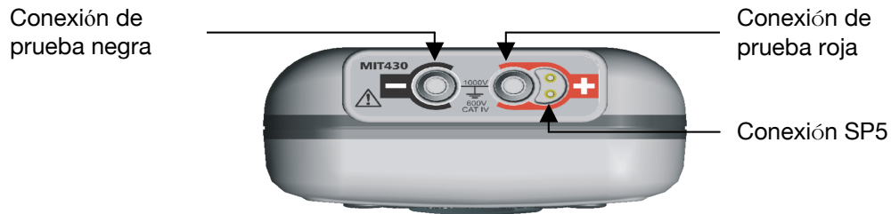
Figura 2, Conexiones de prueba
