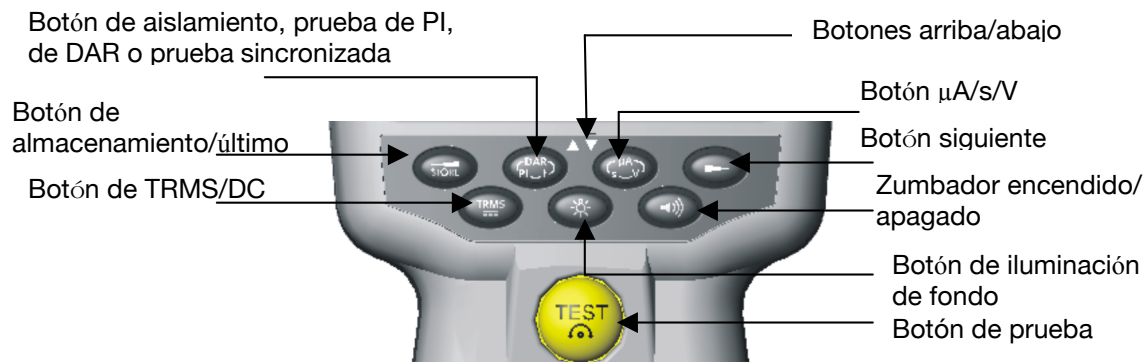
Figura 4, Botones de función (Imagen de MIT430)
