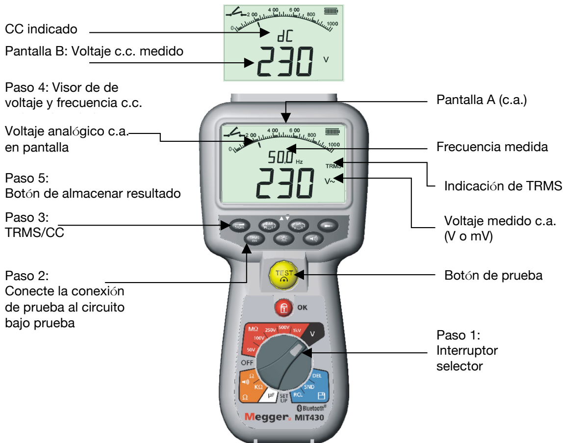
Figura 5, Medición de voltaje y de frecuencia
