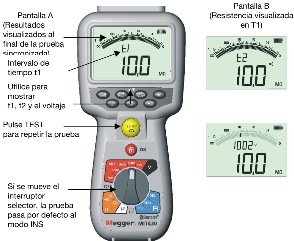
Figura 8, Prueba de aislamiento – modo sincronizado
