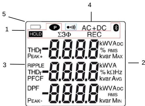
Figure 4 : l’afficheur
