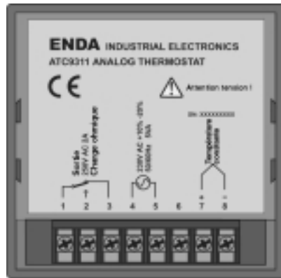
schéma de branchement (3) ATC9311
