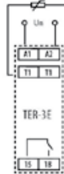
Sonde externe
