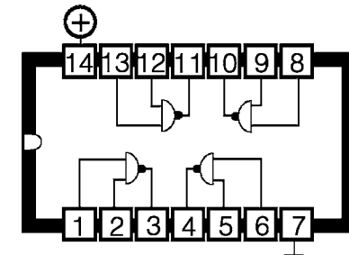
Quatre portes NAND avec 2 entrées
