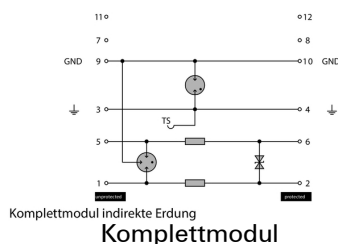
Komplettmodul
